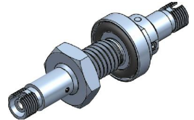
Fiber Optic Feedthrough Type M10 MINI
